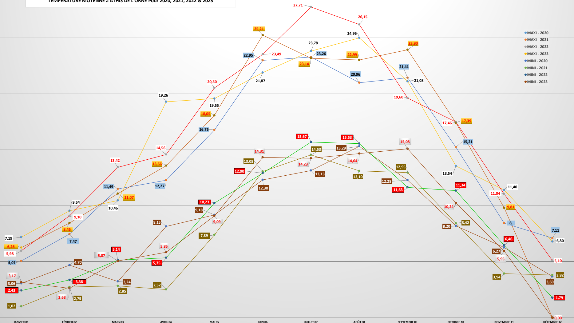
TEMPÉRATURE MOYENNE à ATHIS DE L'ORNE Pour 2020, 2021, 2022 & 2023
